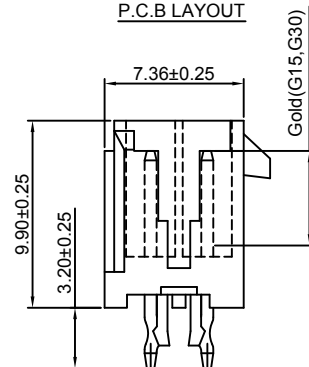
P.C.B LAYOUT
